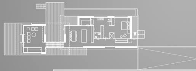
VERDIEPING
